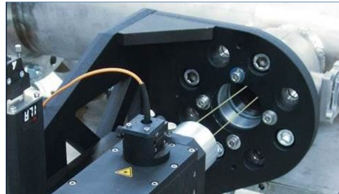
LDV-Sonde im Messzustand
